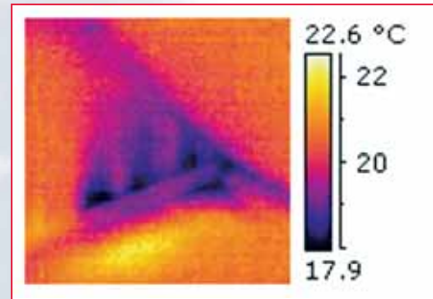
Thermogramm bei Unterdruck während einer BlowerDoor-Messung: Die Leckagen in der Gebäudehülle werden deutlich sichtbar.
